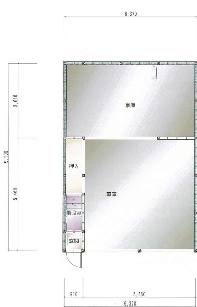
平面詳細図 1階
